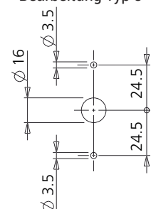
Bearbeitung Typ 3
