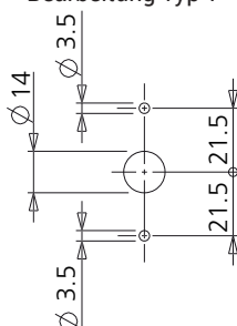
Bearbeitung Typ 1
