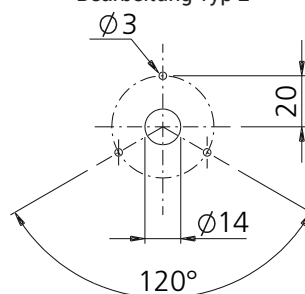
Bearbeitung Typ 2
