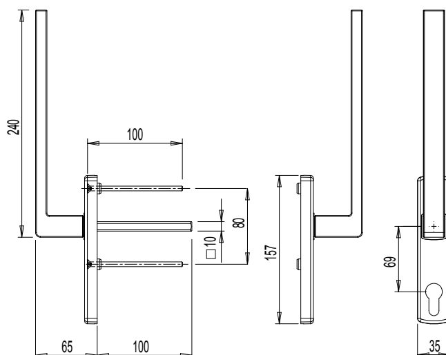
Maße Steckgriff KORA L240 KEY CP -I80
