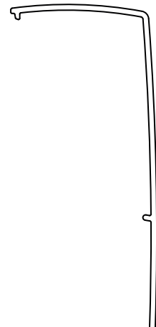
09771 (Einzelprofil)
