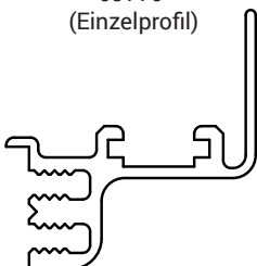
09770 (Einzelprofil)
