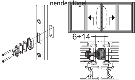
Montage Schließstelle für in entgegengesetzte Richtung öffnende Flügel
