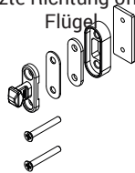
Montage verstellbare Schließstelle 13÷25 mm
