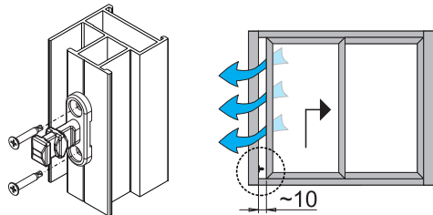
Montage Schließstelle mit Mikrobelüftung
