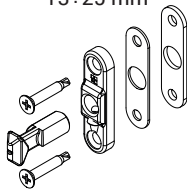
Verstellbare Schließstelle 13÷25 mm
