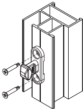
Montage feste Schließstelle
