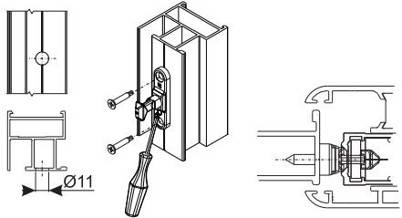
Montage verstellbare Schließstelle 13÷25 mm
