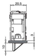
Flache Frontseite
