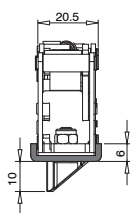
U-förmiges Frontelement
