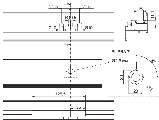
Type A: machining
