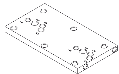
Plantilla de mecanizado perfiles art. 03218
