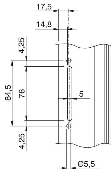
Mecanizado distancia entre ejes 84,5 mm
