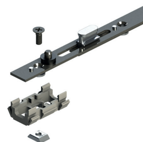
Fijación con expansión (A2)
