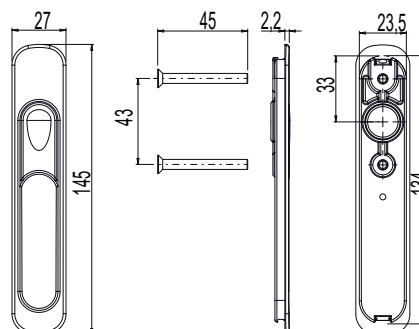
Dimensiones tirador
