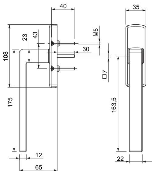
Dimensiones
