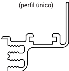
09770 (perfil único)
