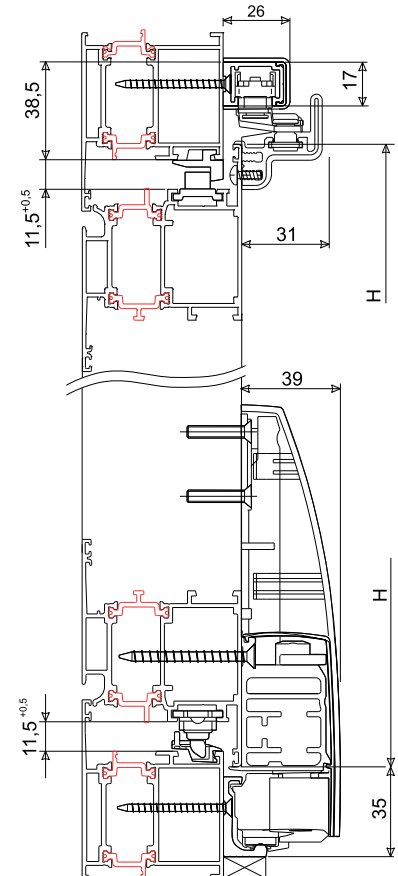
09771 (perfil único)
