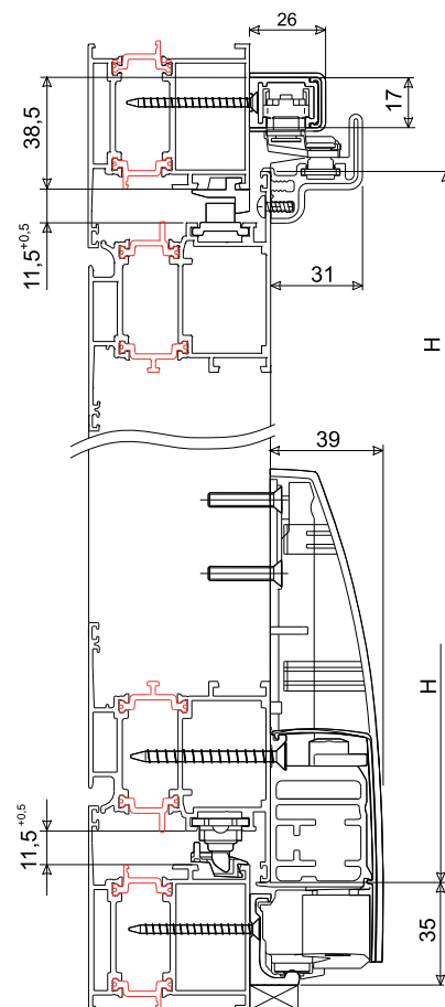
Sección aplicación
