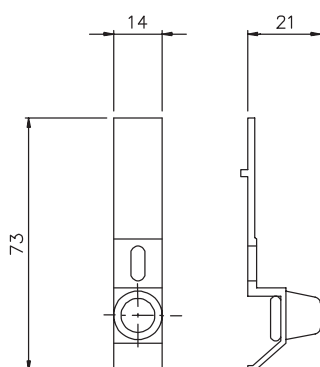
Tapón superior
