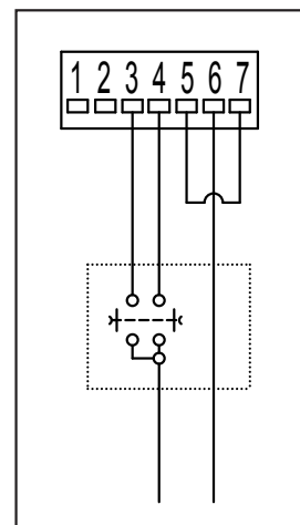
Schéma de câblage
