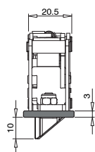
Frontale piatto
