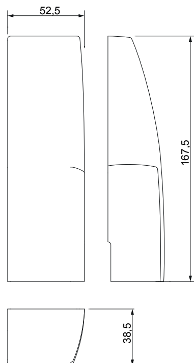
Tampas cód. 09775
