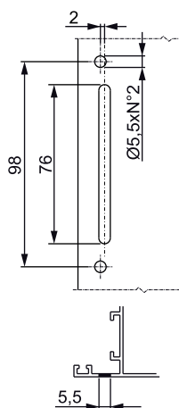
Usinagem do entre-eixo de 98 mm
