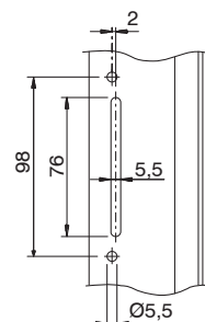
Usinagem do entre-eixo de 98 mm
