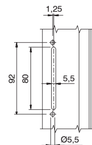
Usinagem do entre-eixo de 92 mm
