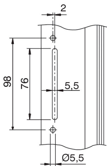
Usinagem do entre-eixo de 98 mm
