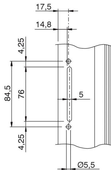
Usinagem do entre-eixo de 84,5 mm
