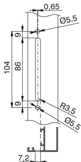
Usinagem do entre-eixo de 104 mm
