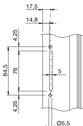
Usinagem do entre-eixo de 84,5 mm
