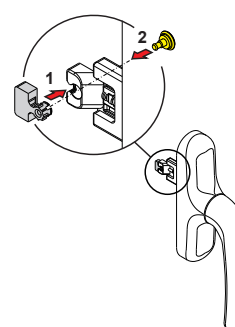
D3 - Montagem de calços para anti falsa mecanismo
