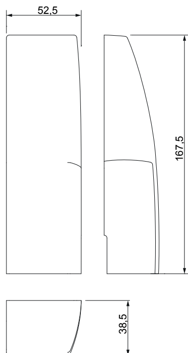
Заглушки защитного профиля из Арт. 09775
