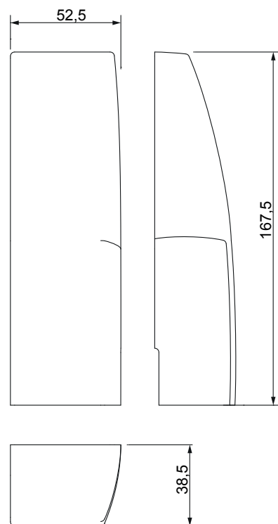
Заглушки защитного профиля из Арт. 09775
