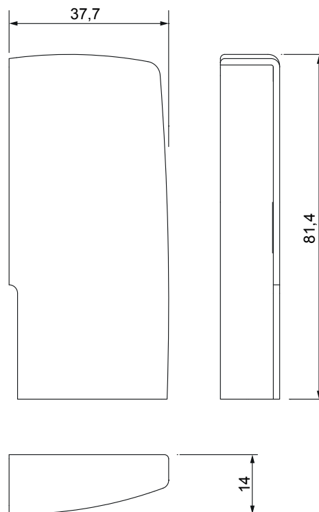
Заглушки защитного профиля из Арт. 09774
