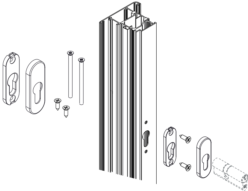
Арт. 04096 Последовательность монтажа Арт. 04096
