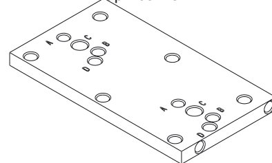
ШАБЛОН ДЛЯ СВЕРЛЕНИЯ ОТВЕРСТИЙ, арт. 03218
