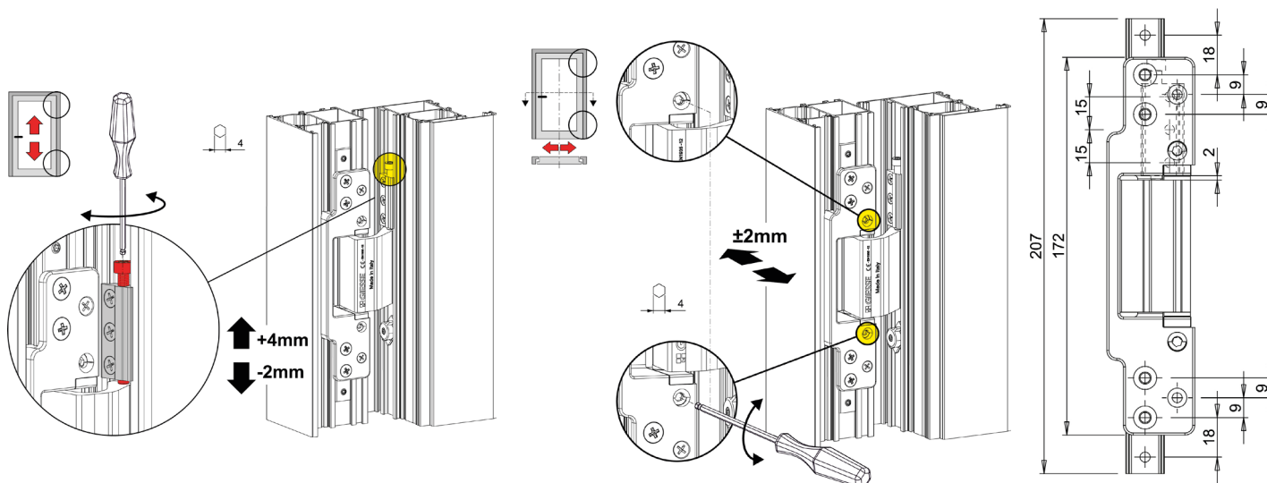
Регулировка створки по высоте
