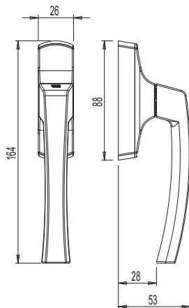
Размеры арт. 01401
