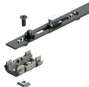
Расширяющееся крепление (A2)
