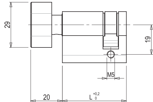
Размеры ручки типа 1
