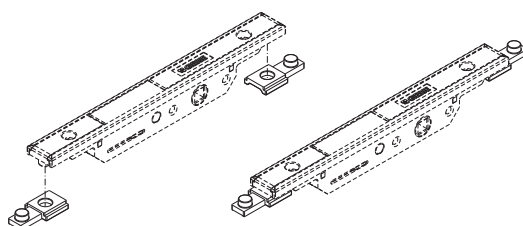
Сборка с механизмом 0102001
