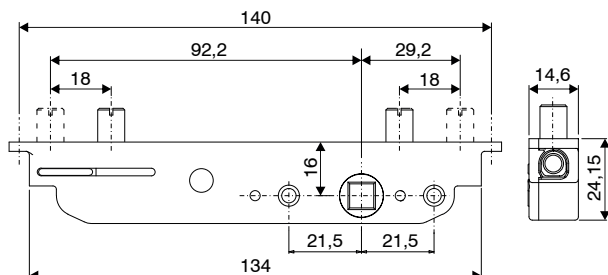
Тип С: размеры
