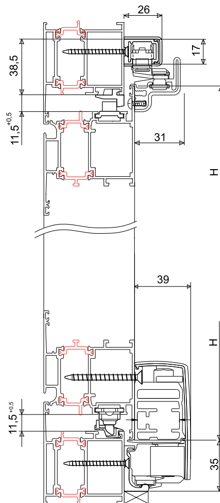
09771 (единый профиль)
