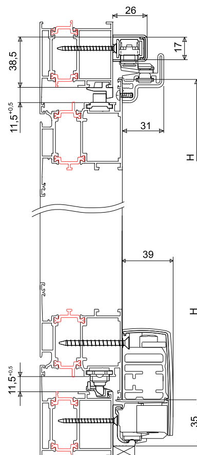
09771 (единый профиль)
