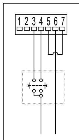
Схема кабельного подключения
